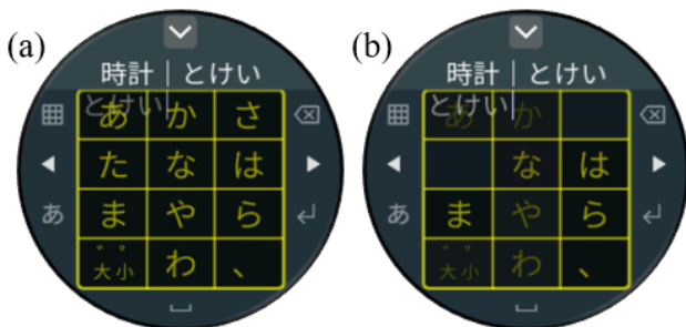
図6 段階的な透明化. a)初期はキートップをしっかりと見える程度の透明度で表示. b)入力ミスの頻度が少ないキーは透明度を上げていき,最終的に完全に透明な状態になる.
